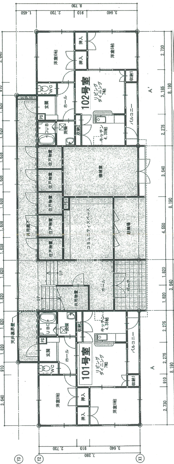
定住促進住宅【東棟】平面図
