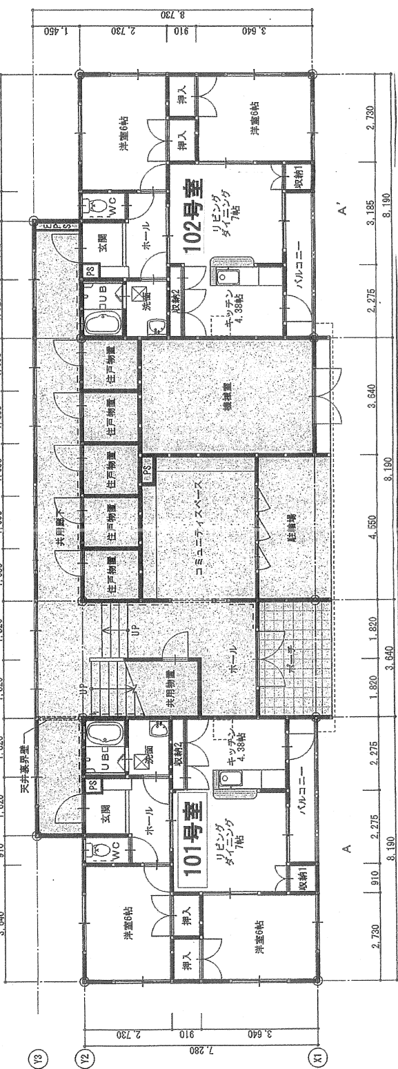
定住促進住宅【東棟】平面図
